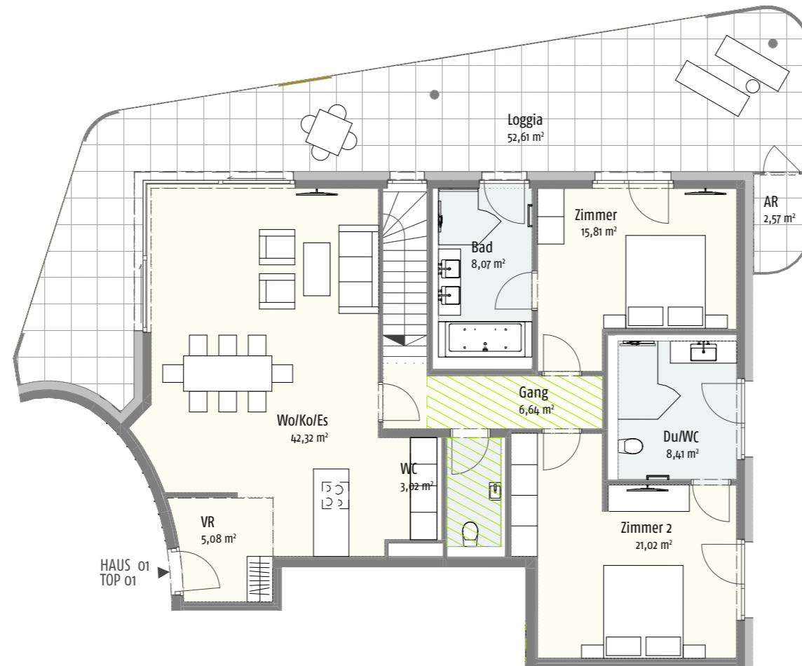
Erdgeschoss
